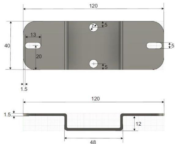
Abbildung 3. Sensormontageadapter für TAC-B 4G
