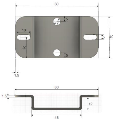
Abbildung 2. Sensormontageadapter für TAC-B WP
